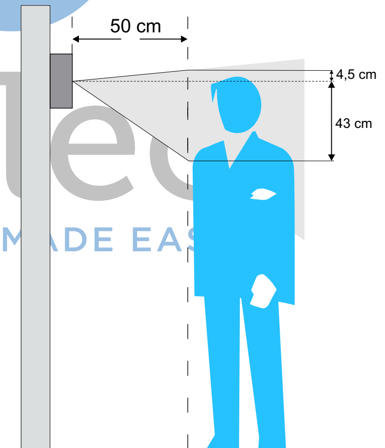
Stelbare camera maximaal omlaag gericht
