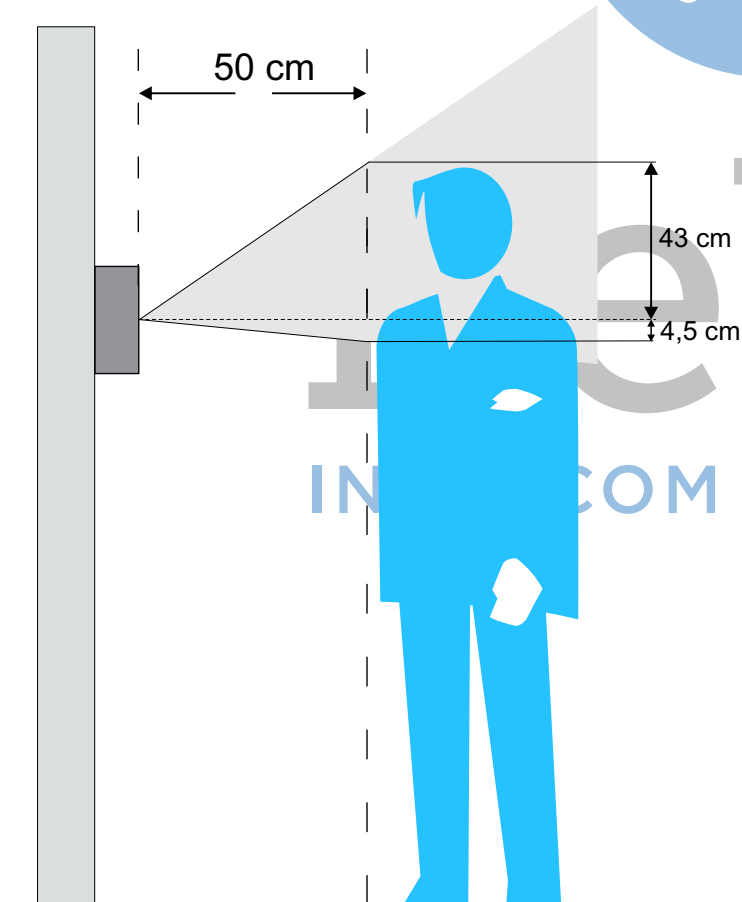
Stelbare camera maximaal omhoog gericht
