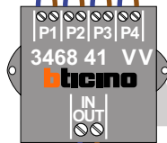
Max. 100 meter systeem- kabel tot laatste videofoon
