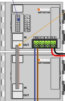
DEURSTATION S-131A
